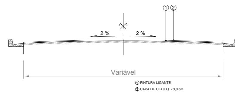
SEÇÃO TRANSVERSAL DO RECAPEAMENTO SEM / ESC.
