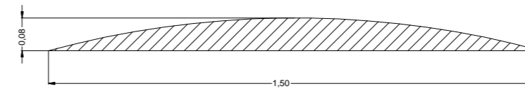
SEÇÃO ONDULAÇÃO TRANSVERSAL TIPO I SEM / ESC.
